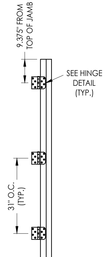
HINGE JAMB
